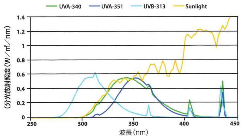
アトラス紫外線蛍光ランプと太陽光との比較 (0.55W/m 2 で制御された分布)
